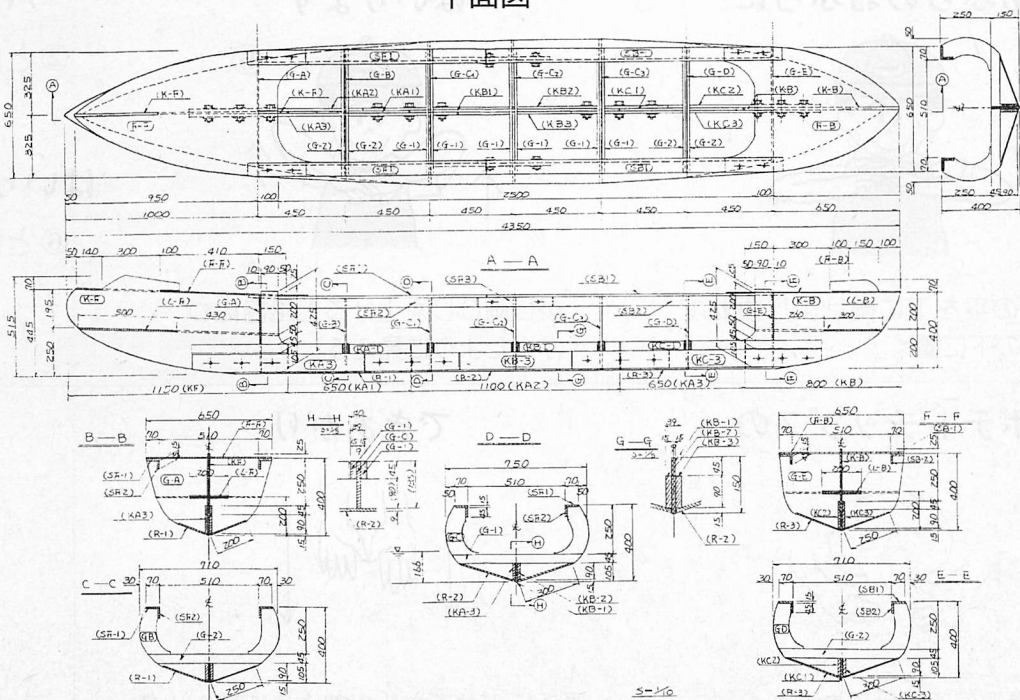
平面図
